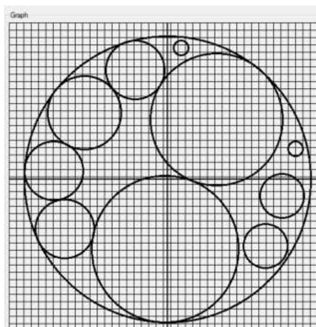
Рис. 2. Локальний мінімум
